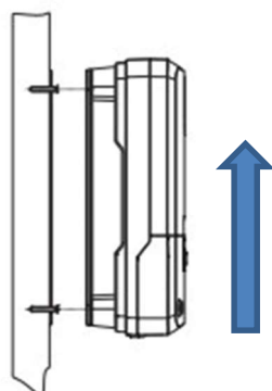
Figura 19. Desmontaje regulador
