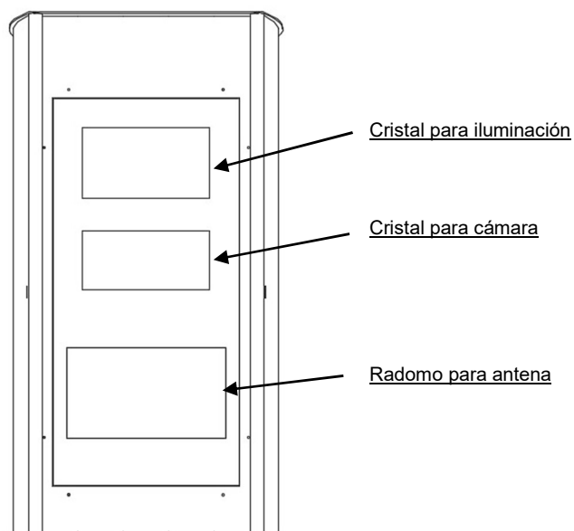
Figura 9. Detalle frontal
