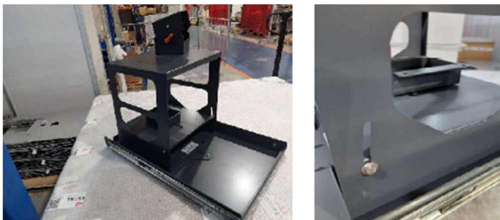
Figura 13. Bandeja extraíble
