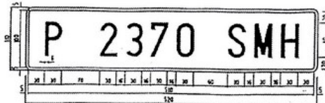
Matricula temporal particular larga Fondo verde. Caracteres blanco mate
