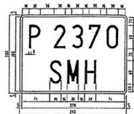
Matricula temporal particular alta Fondo verde. Caracteres blanco mate
