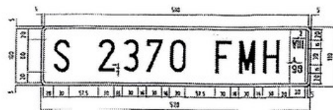
Matricula temporal empresas larga (Vehículos no matriculados) Fondo rojo. Caracteres blanco mate Banda: Fondo blanco. Caracteres rojo mate adhesivos
