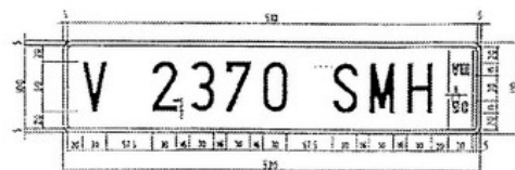
Matricula temporal empresas larga (Vehículos matriculados) Fondo rojo. Caracteres blanco mate Banda: Fondo blanco. Caracteres rojo mate adhesivos
